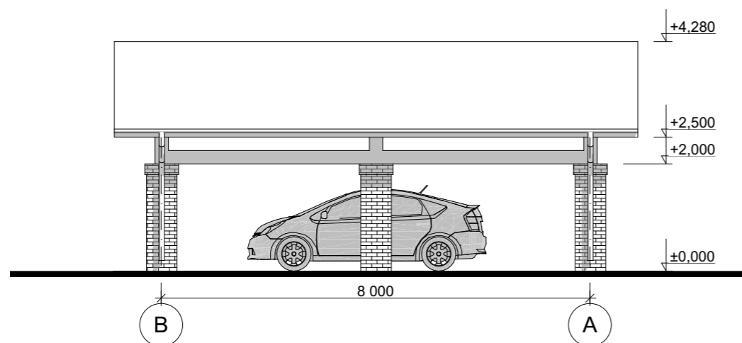
Фасад В-А М 1:100
