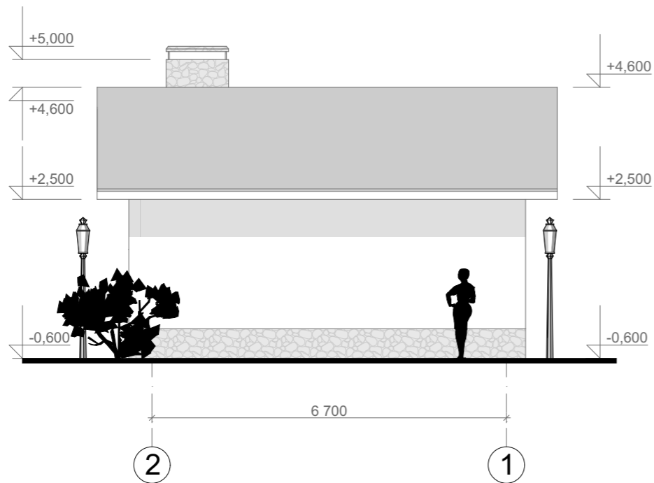
Фасад 2-1 М 1:100
