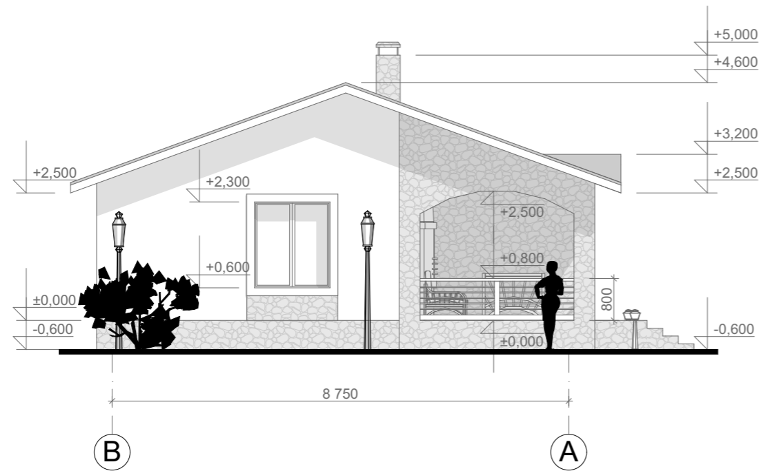
Фасад В-А М 1:100
