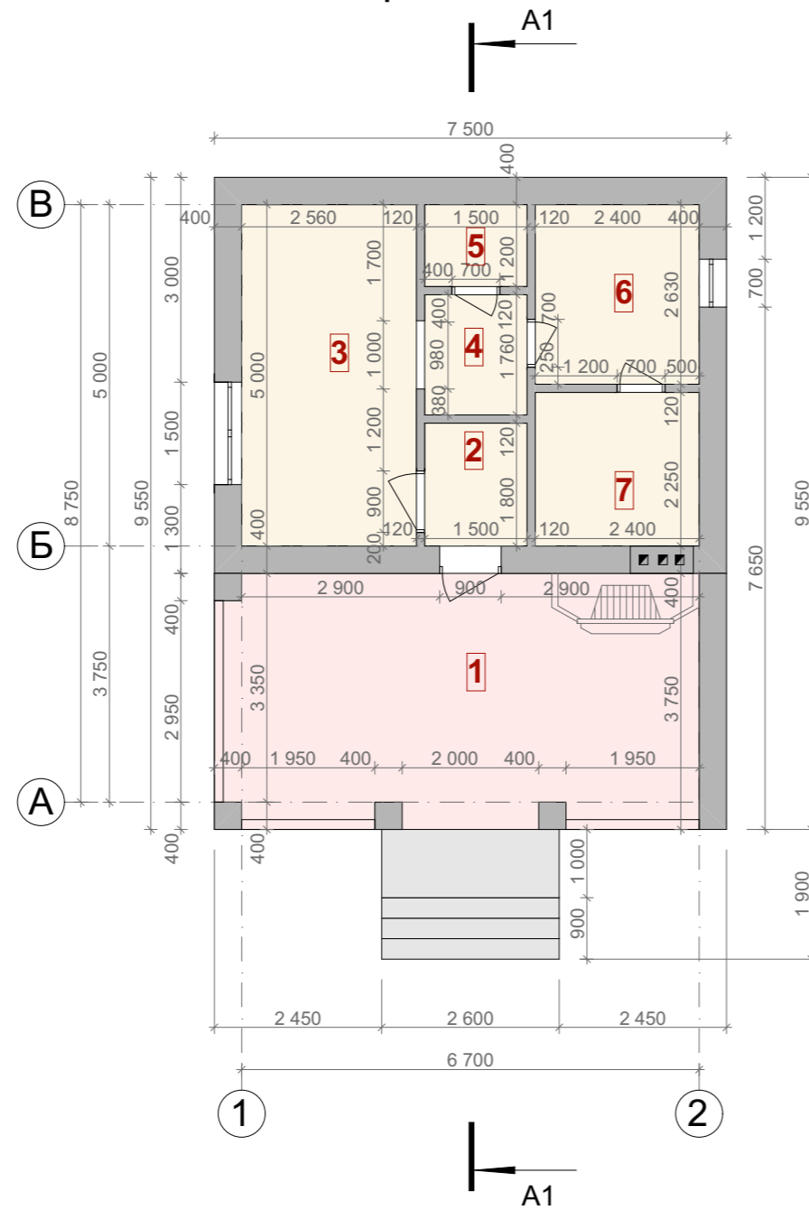
План первого этажа М 1:100
