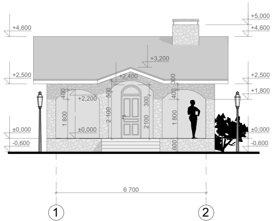
Фасад 1-2 М 1:100
