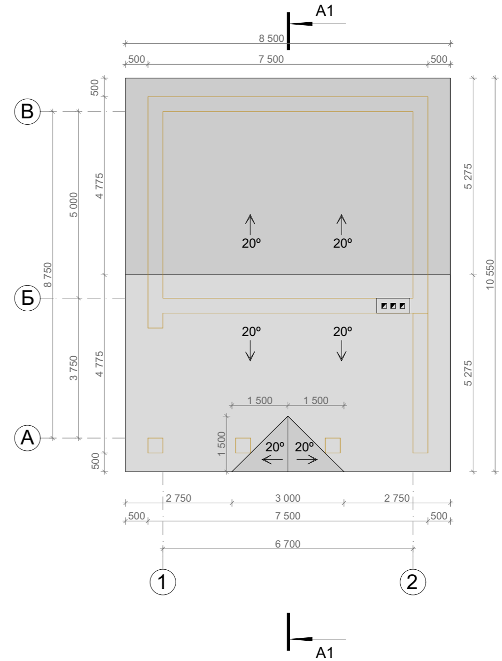
План кровли М 1:100
