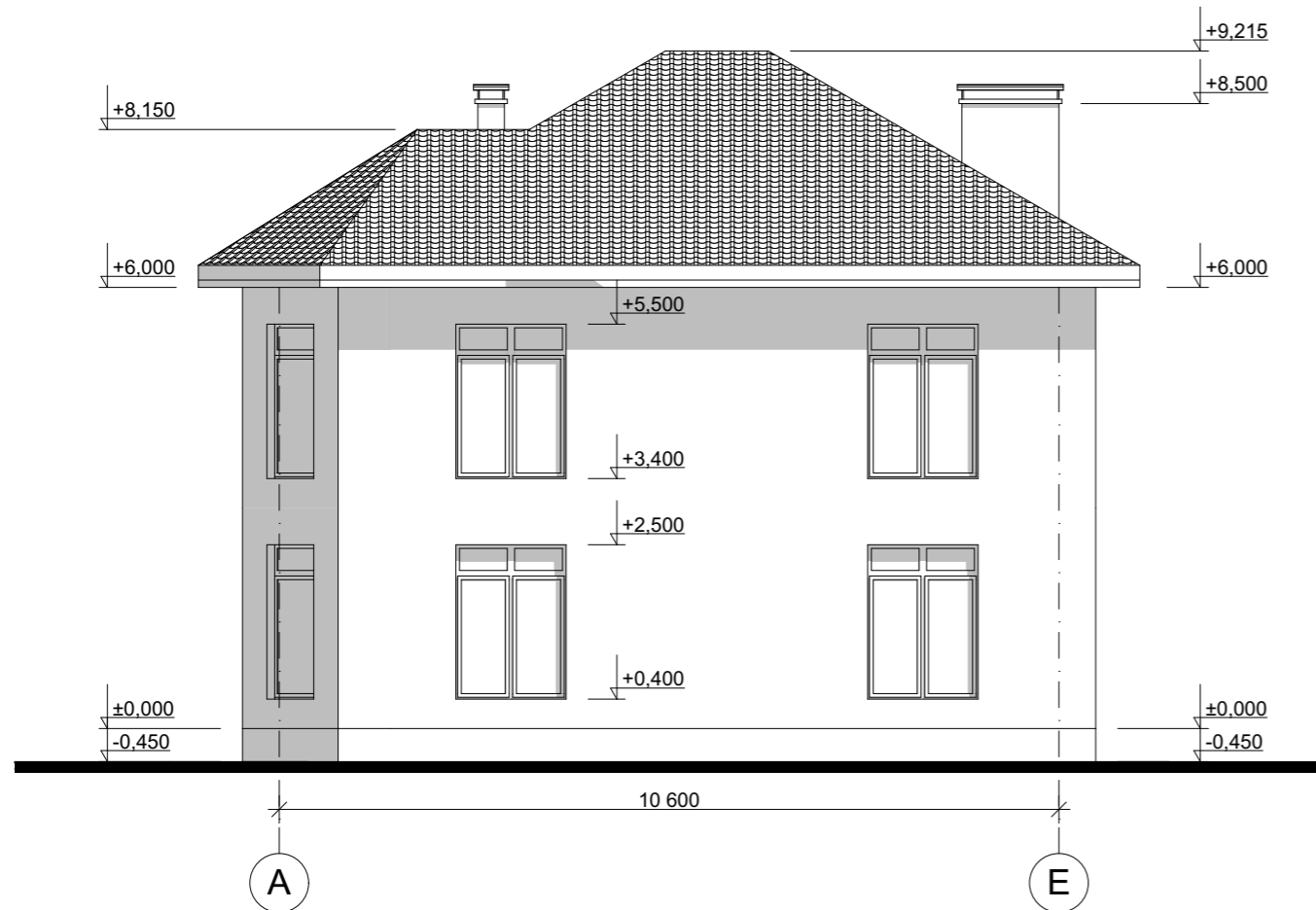
Фасад А-Е М 1:100
