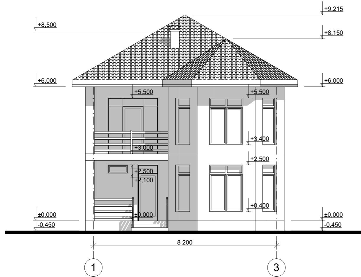
Фасад 1-3 М 1:100
