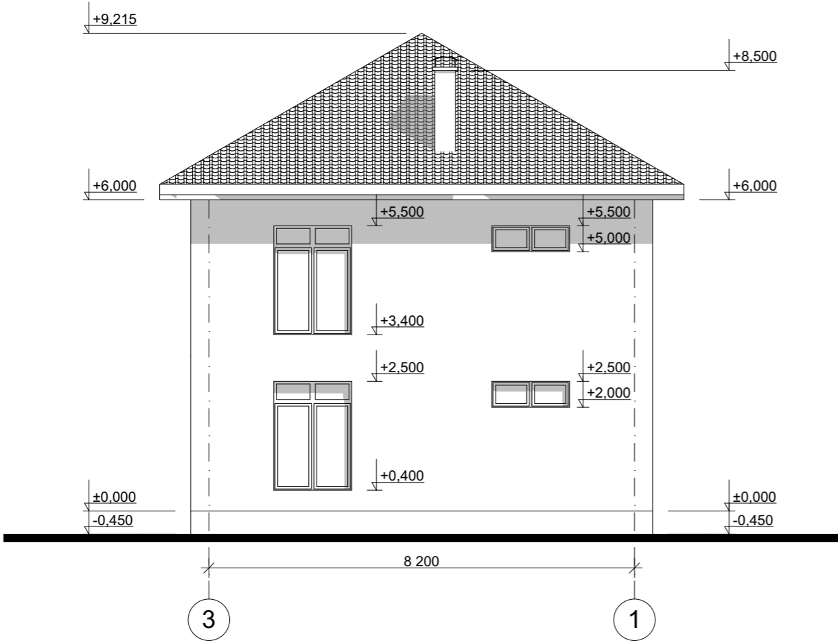
Фасад 3-1 М 1:100
