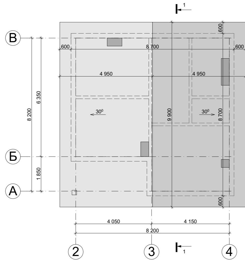
План кровли М 1:100
