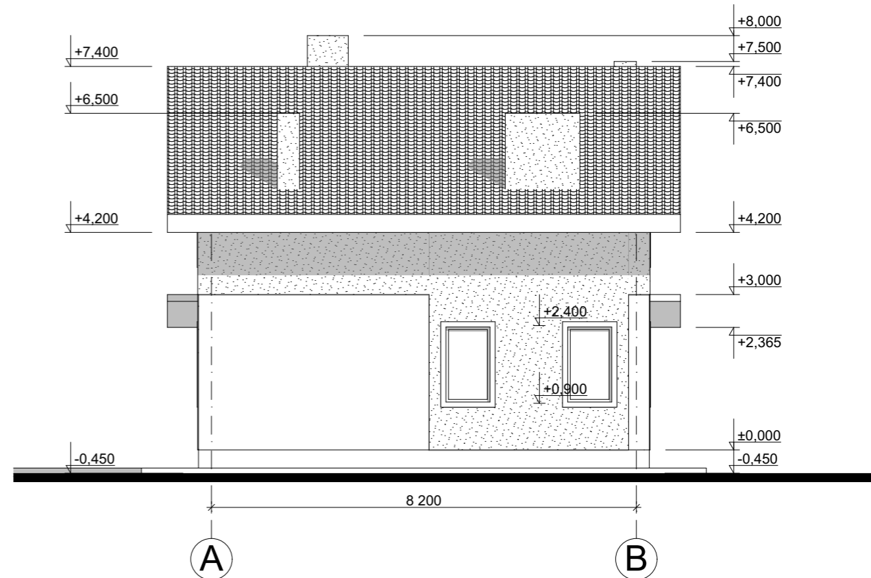
Фасад А-В М 1:100
