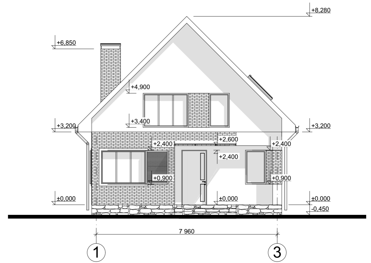
Фасад 1-3 М 1:100
