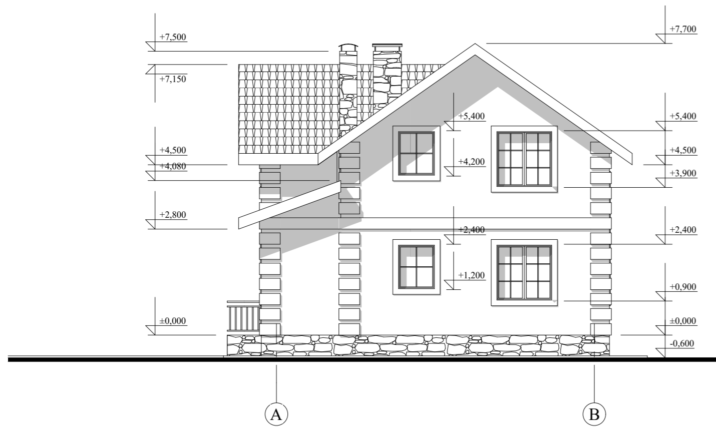
Фасад А-В М 1:100
