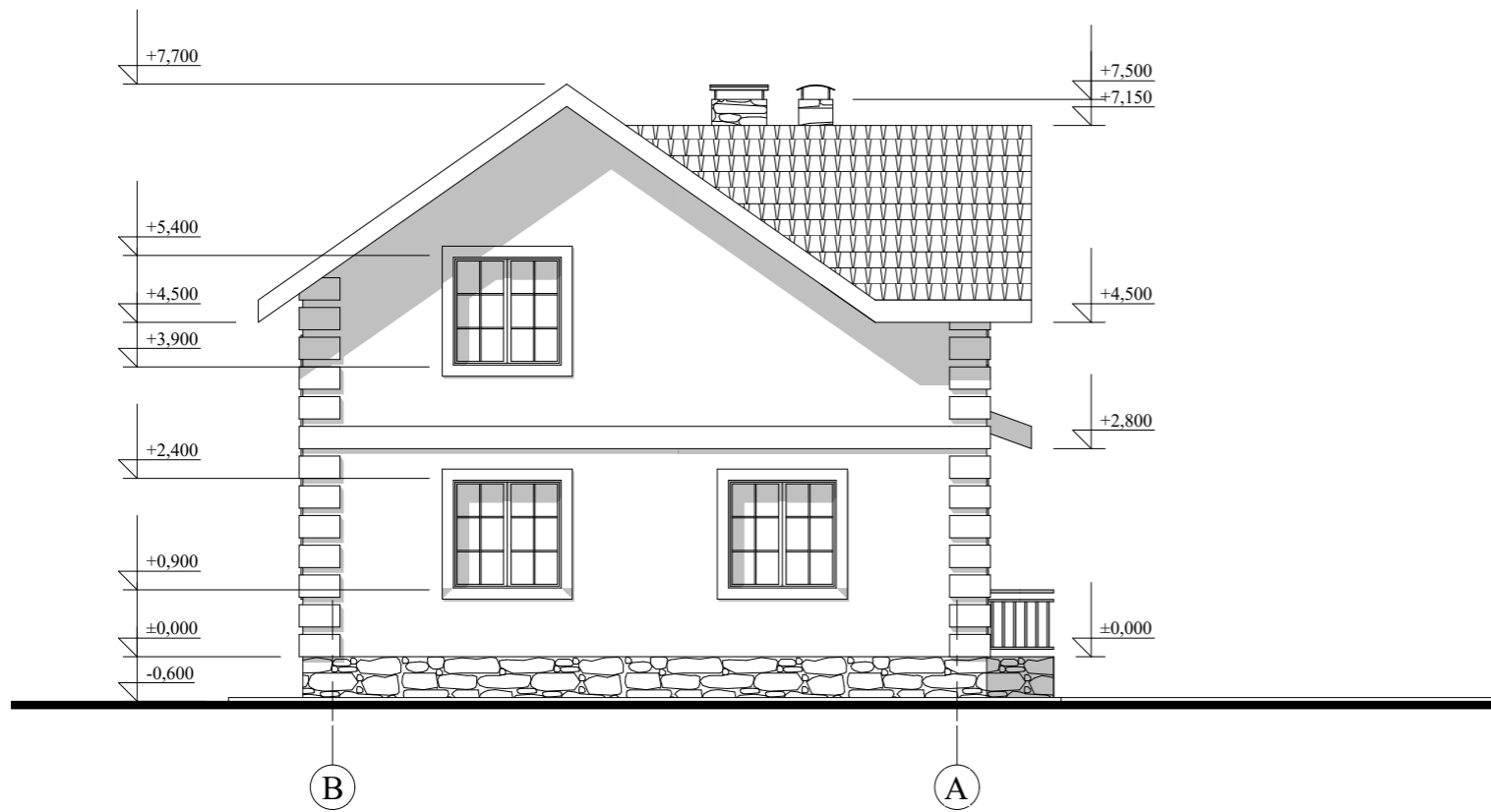
Фасад В-А М 1:100
