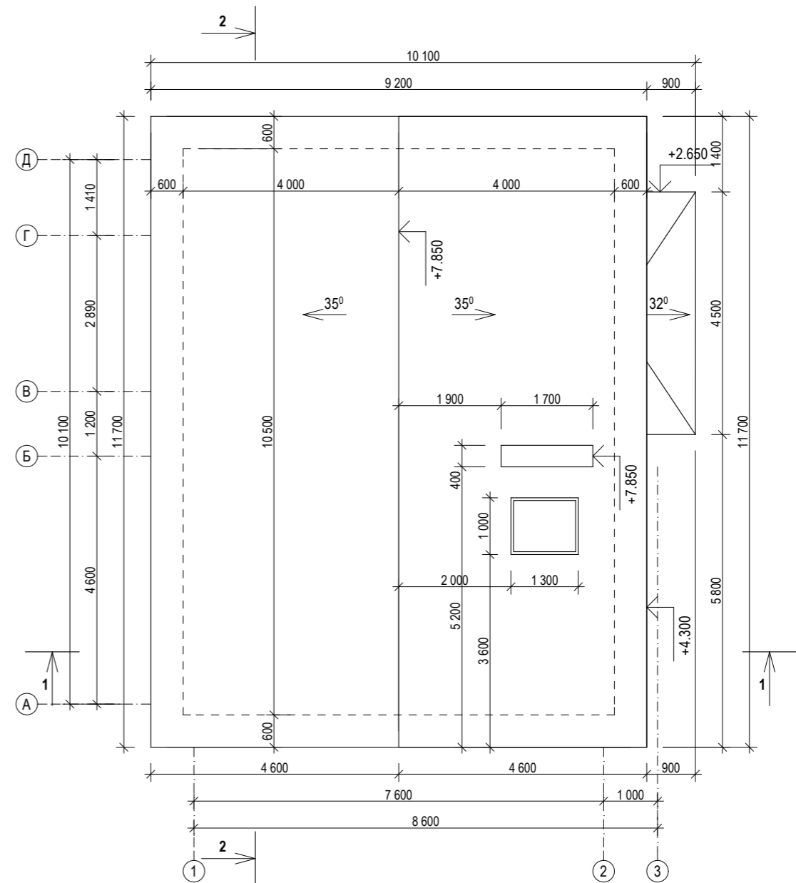
План кровли
