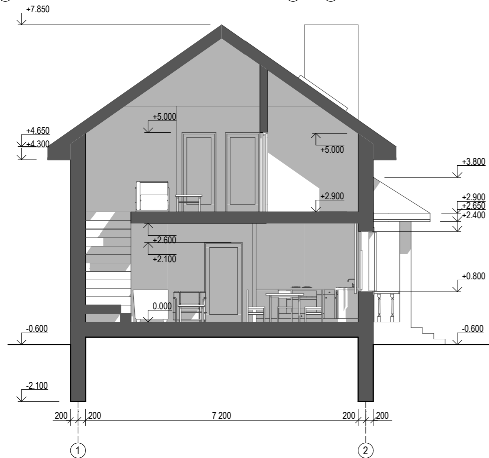
Разрез 1-1
