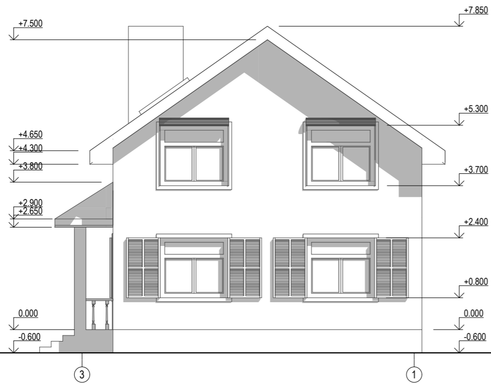
Фасад 3-1
