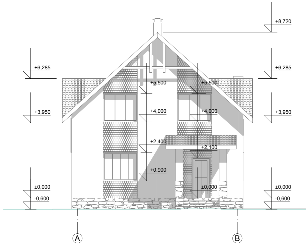
Фасад А-В М 1:100
