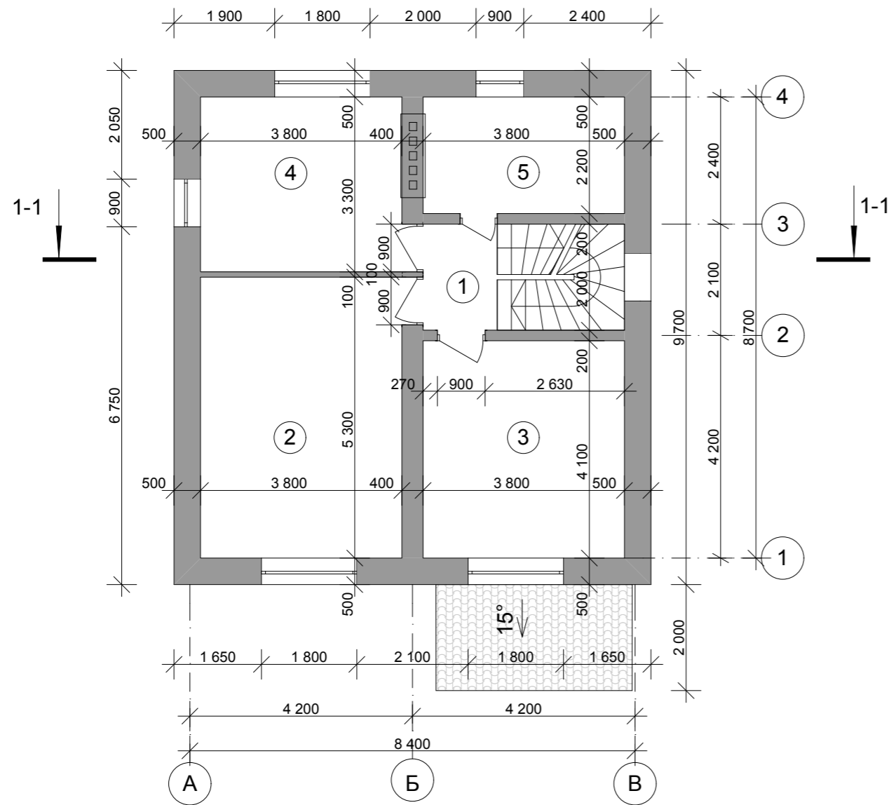
План второго этажа М 1:100
