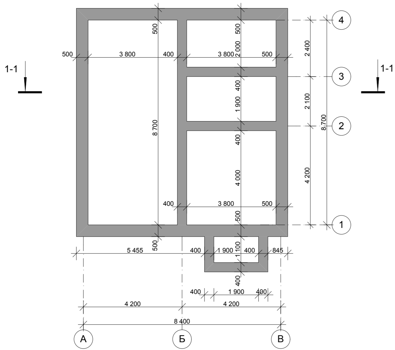
План фундаментов М 1:100
