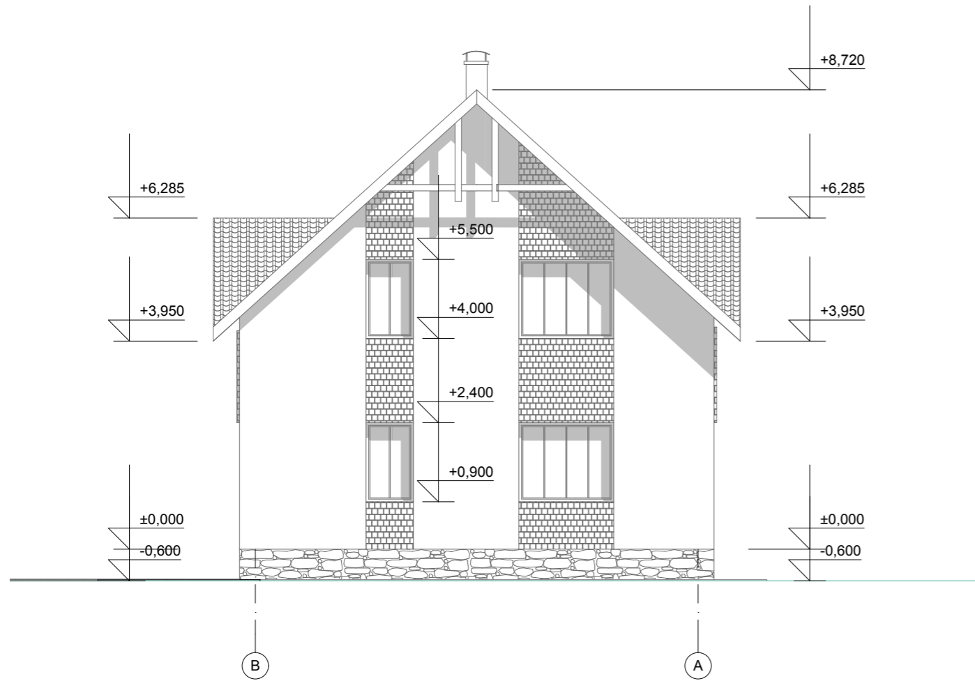
Фасад В-А М:100
