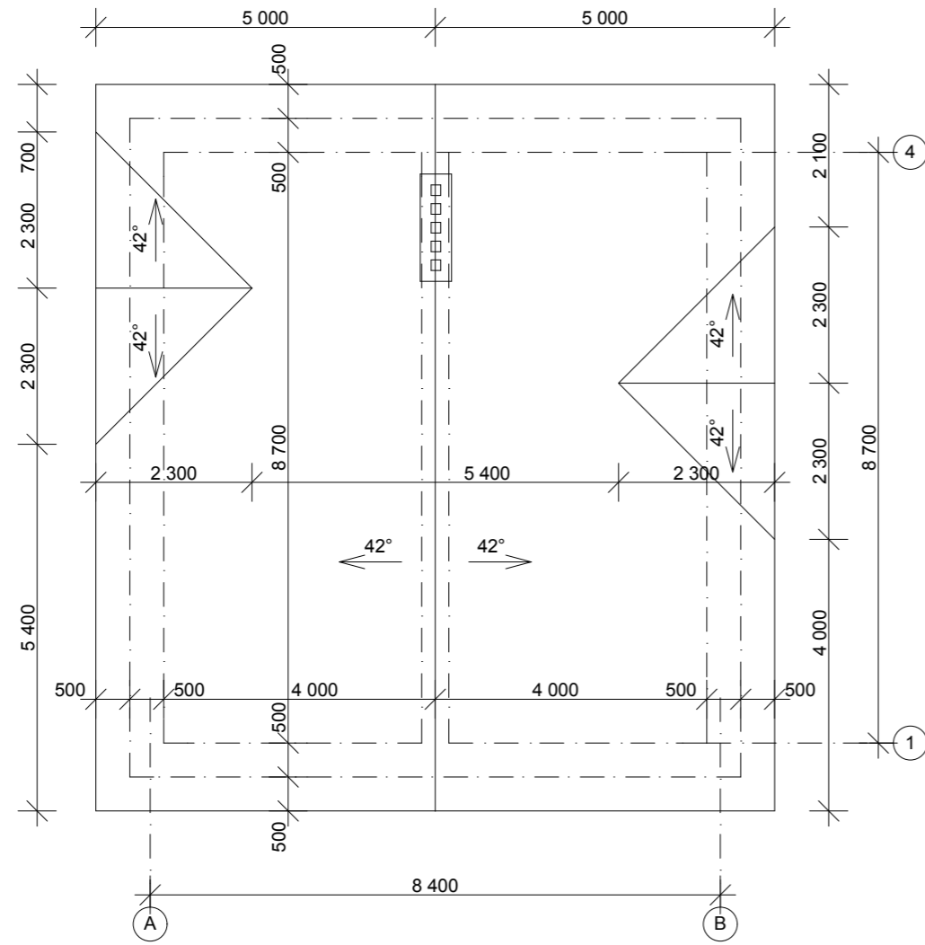
План кровли М 1:100
