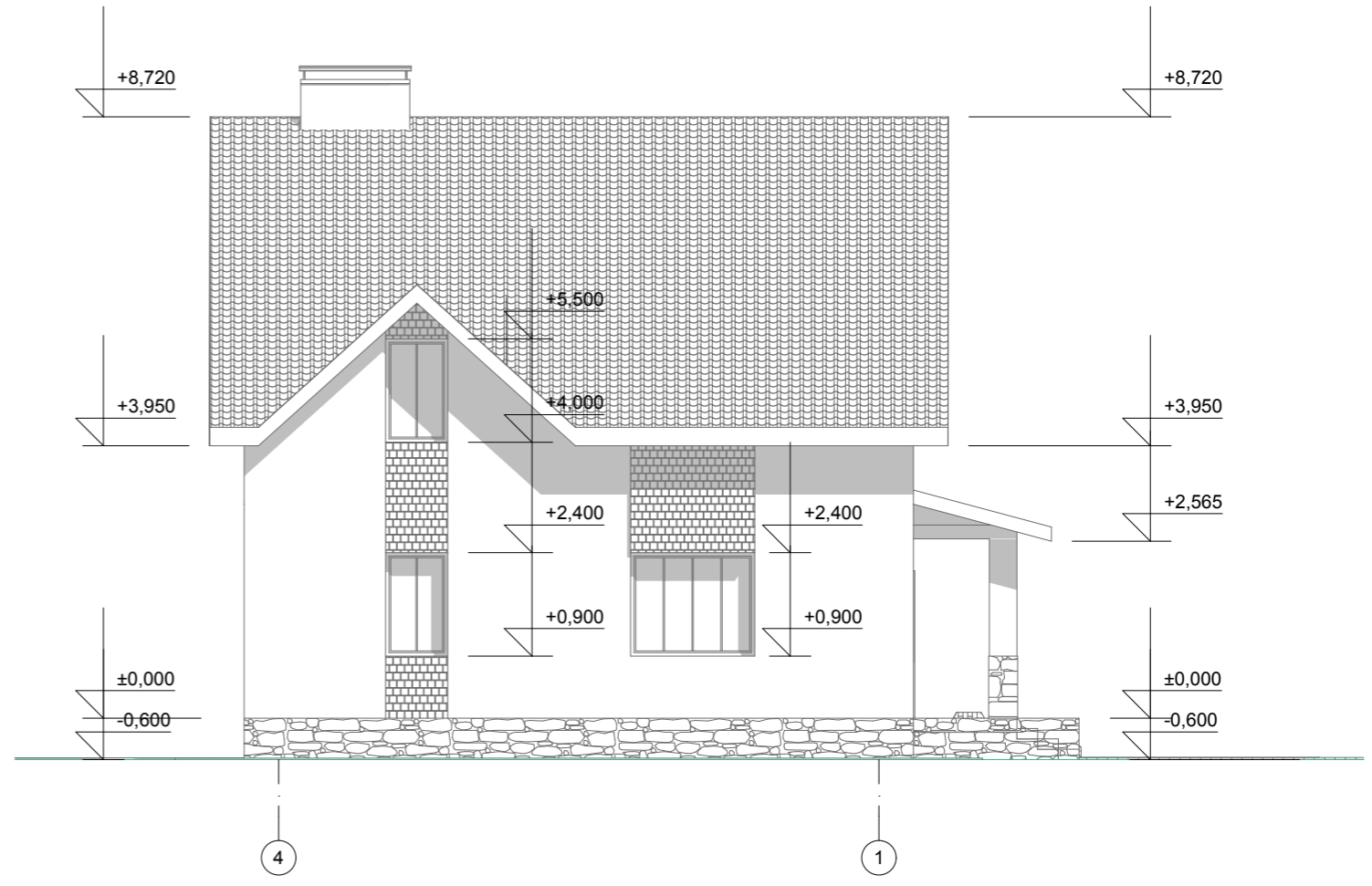
Фасад 4-1 М 1:100
