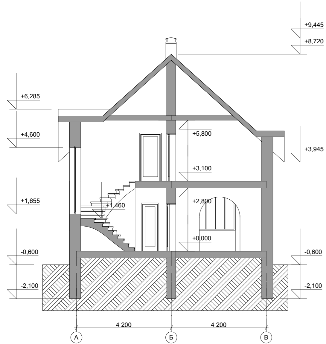
Разрез 1-1 М 1:100
