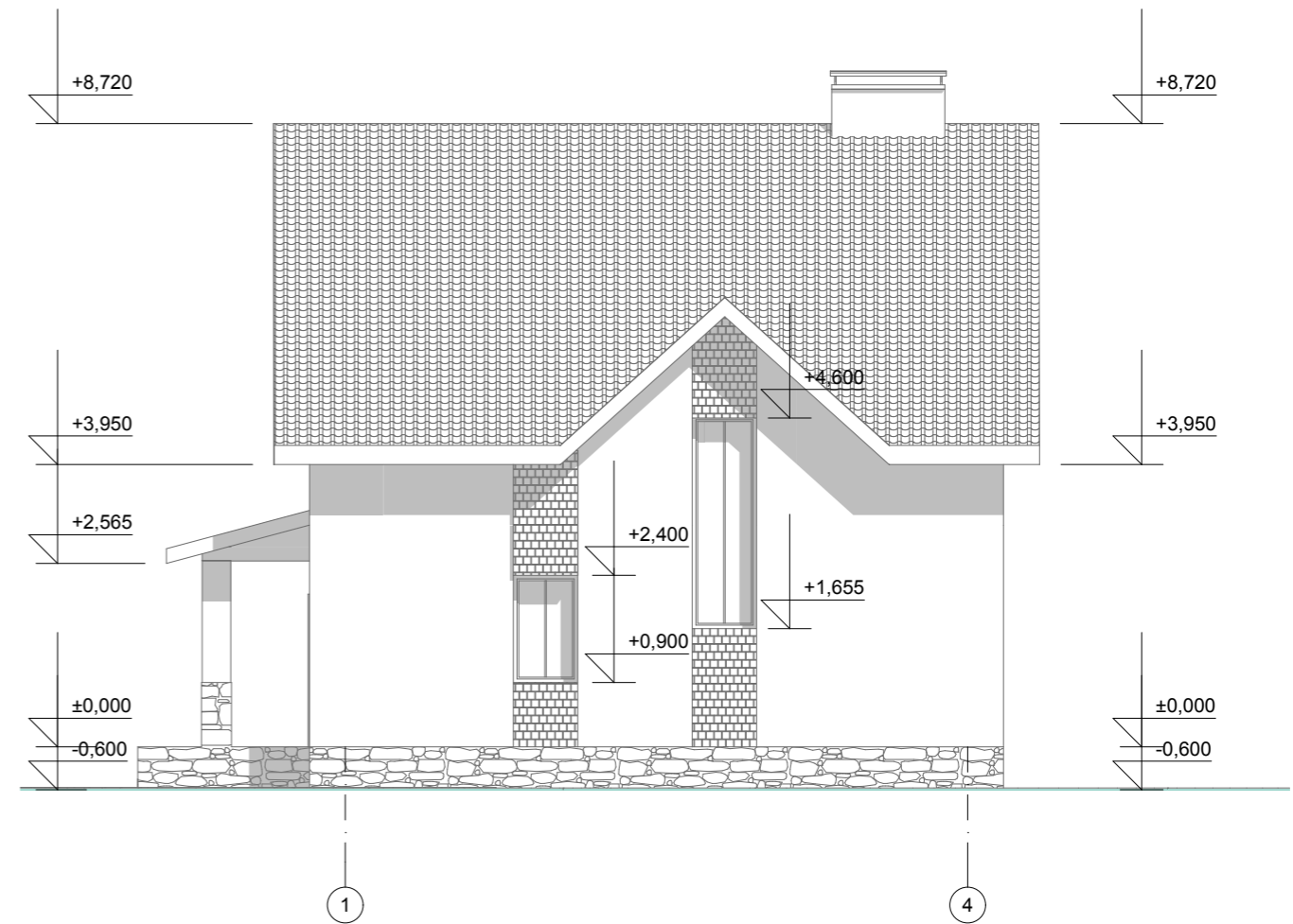
Фасад 1-4 М:100
