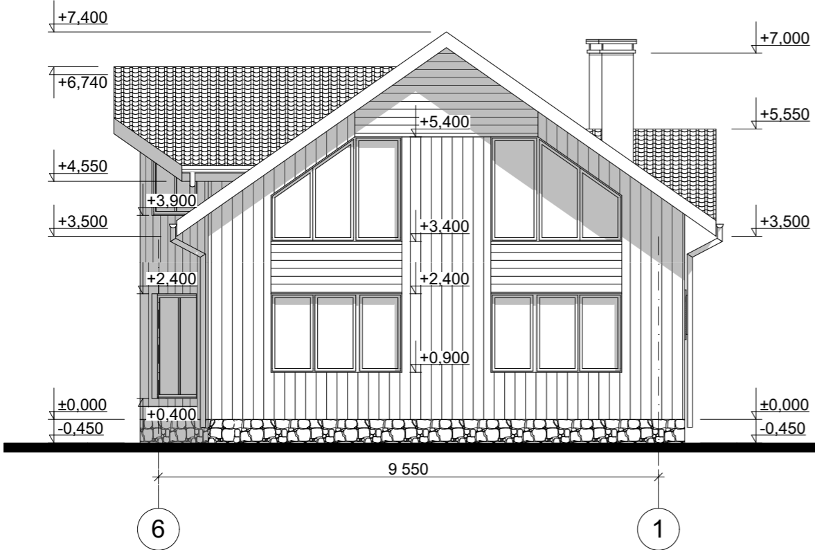
Фасад 6-1 М 1:100
