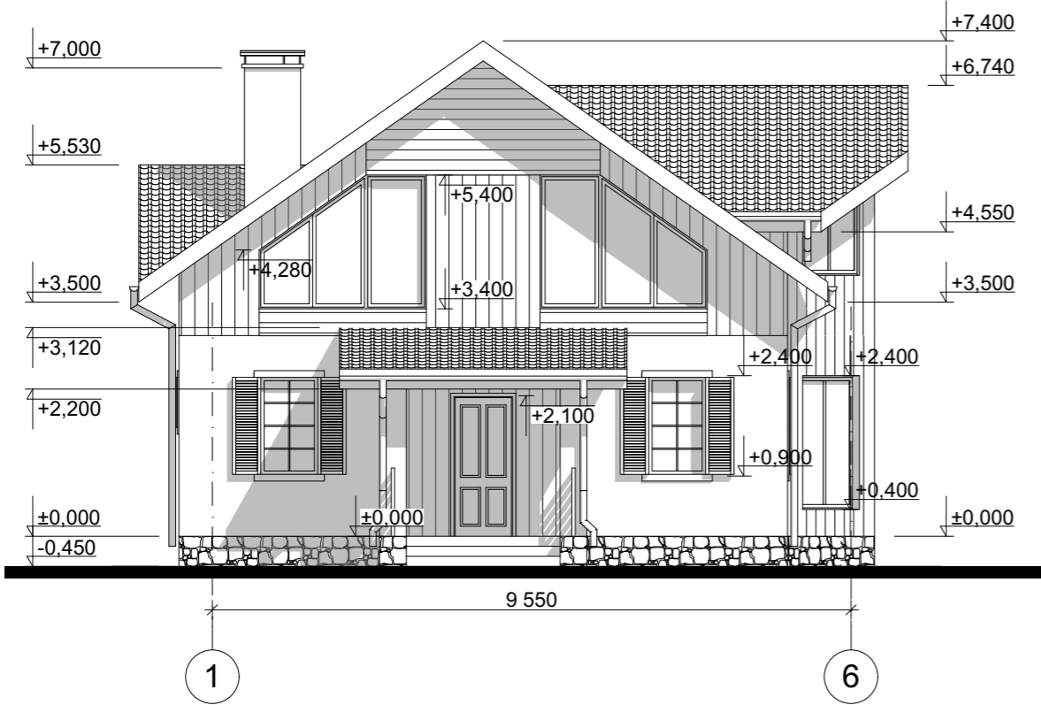
Фасад 1-6 М 1:100
