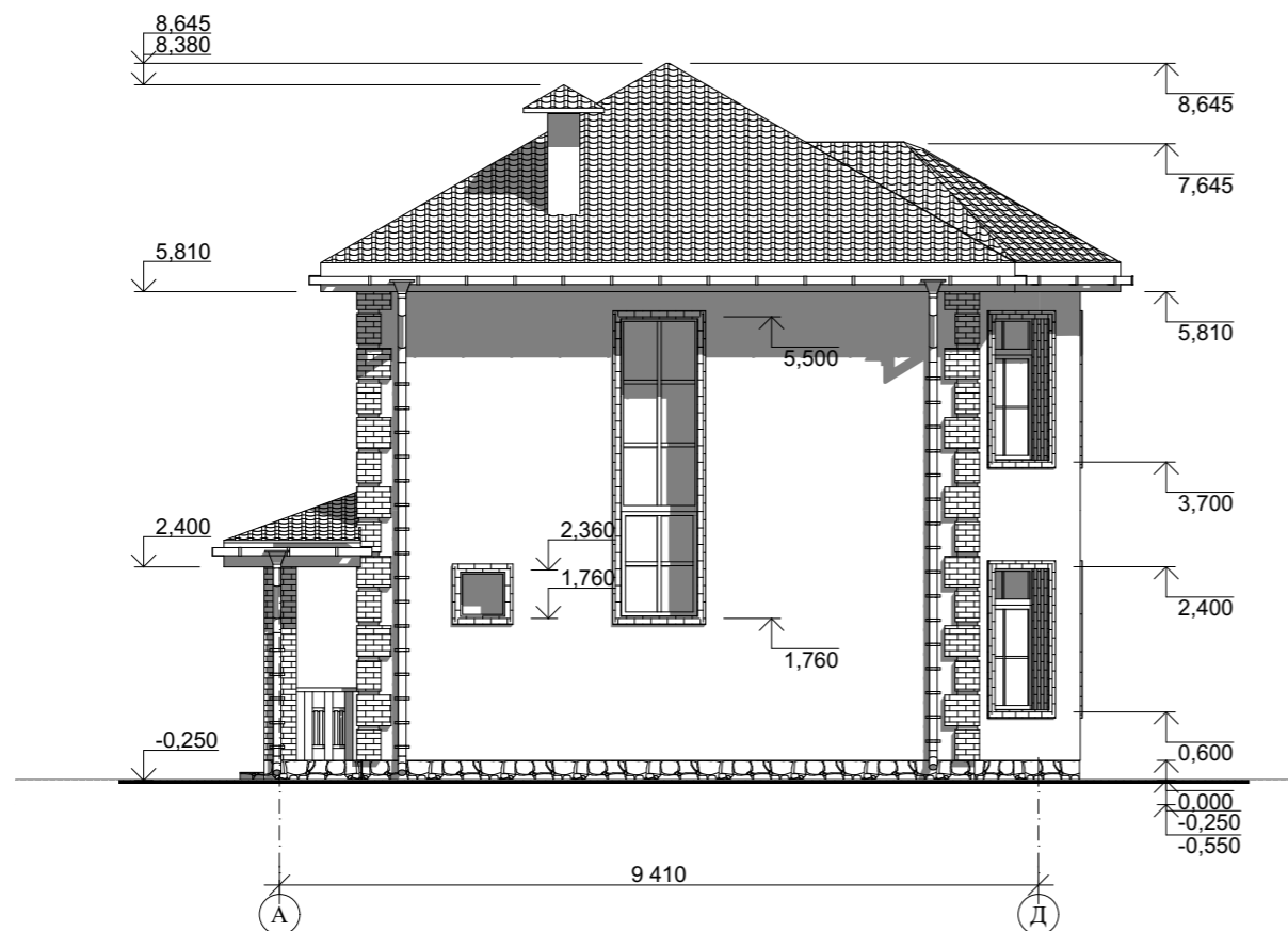
Фасад А-Д М 1:100
