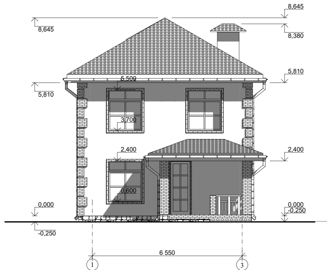
Фасад Д-А М 1:100
