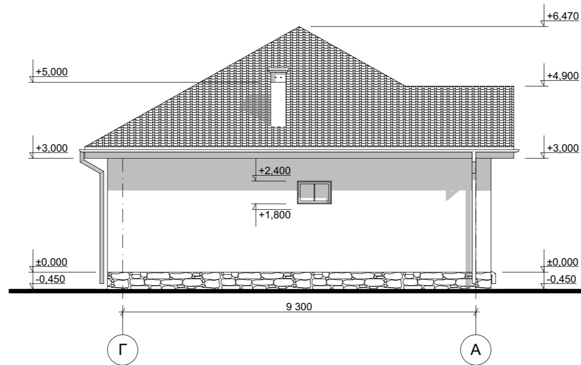
Фасад Г-А М 1:100
