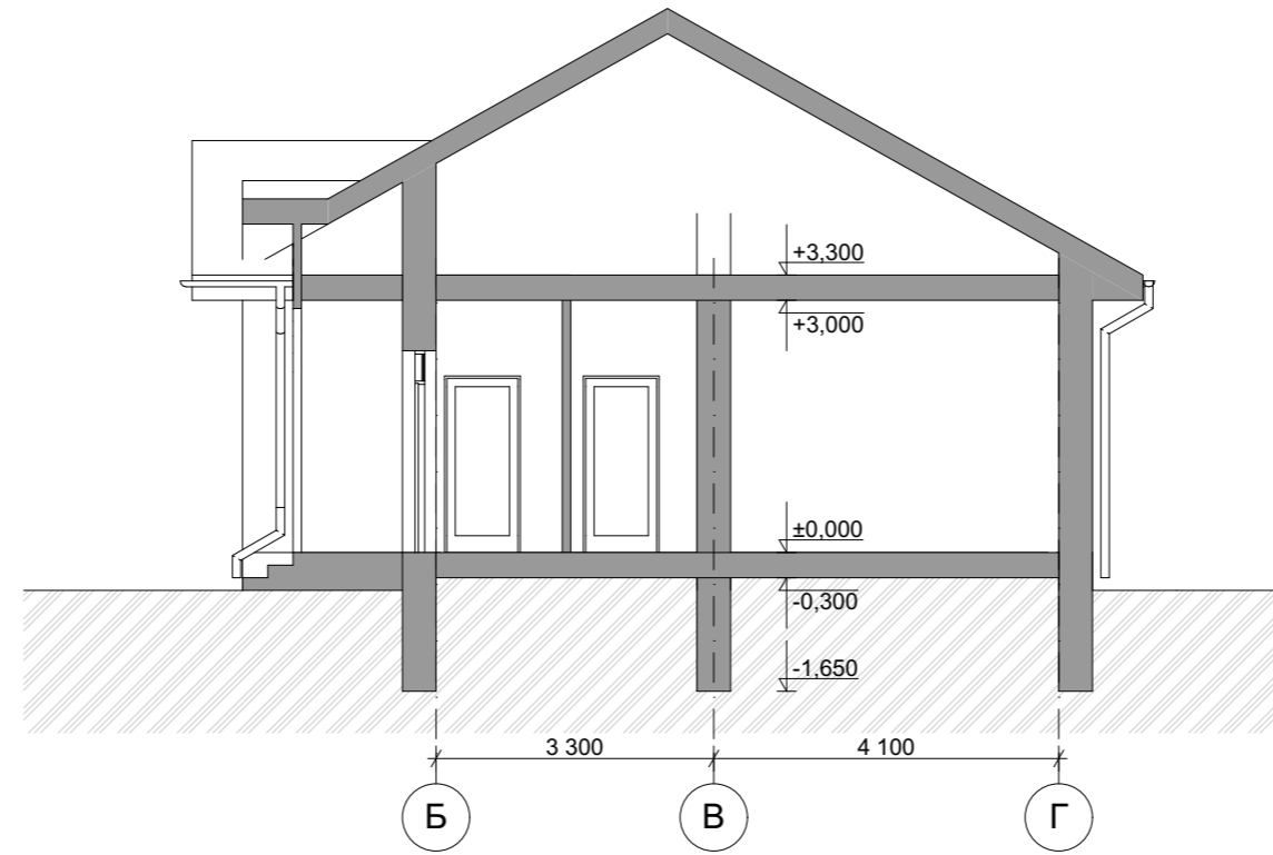
Разрез 1-1 М 1:100
