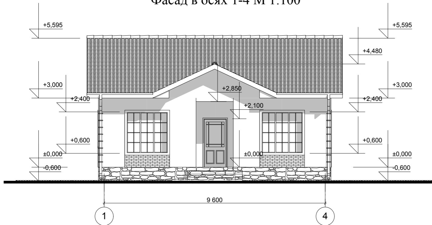
Фасад в осях 1-4 М 1:100
